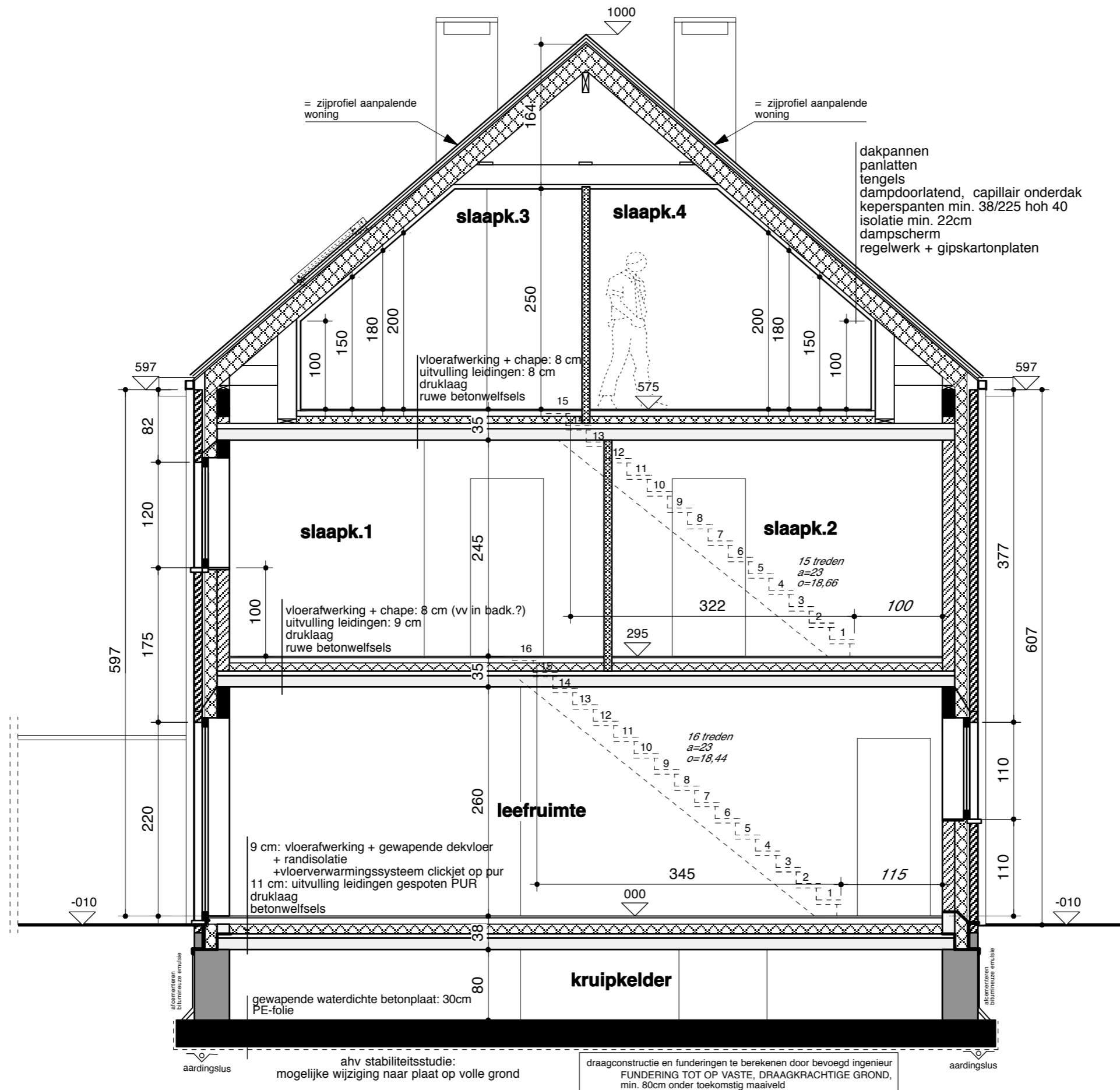
DOORSNEDE A - 1/50
