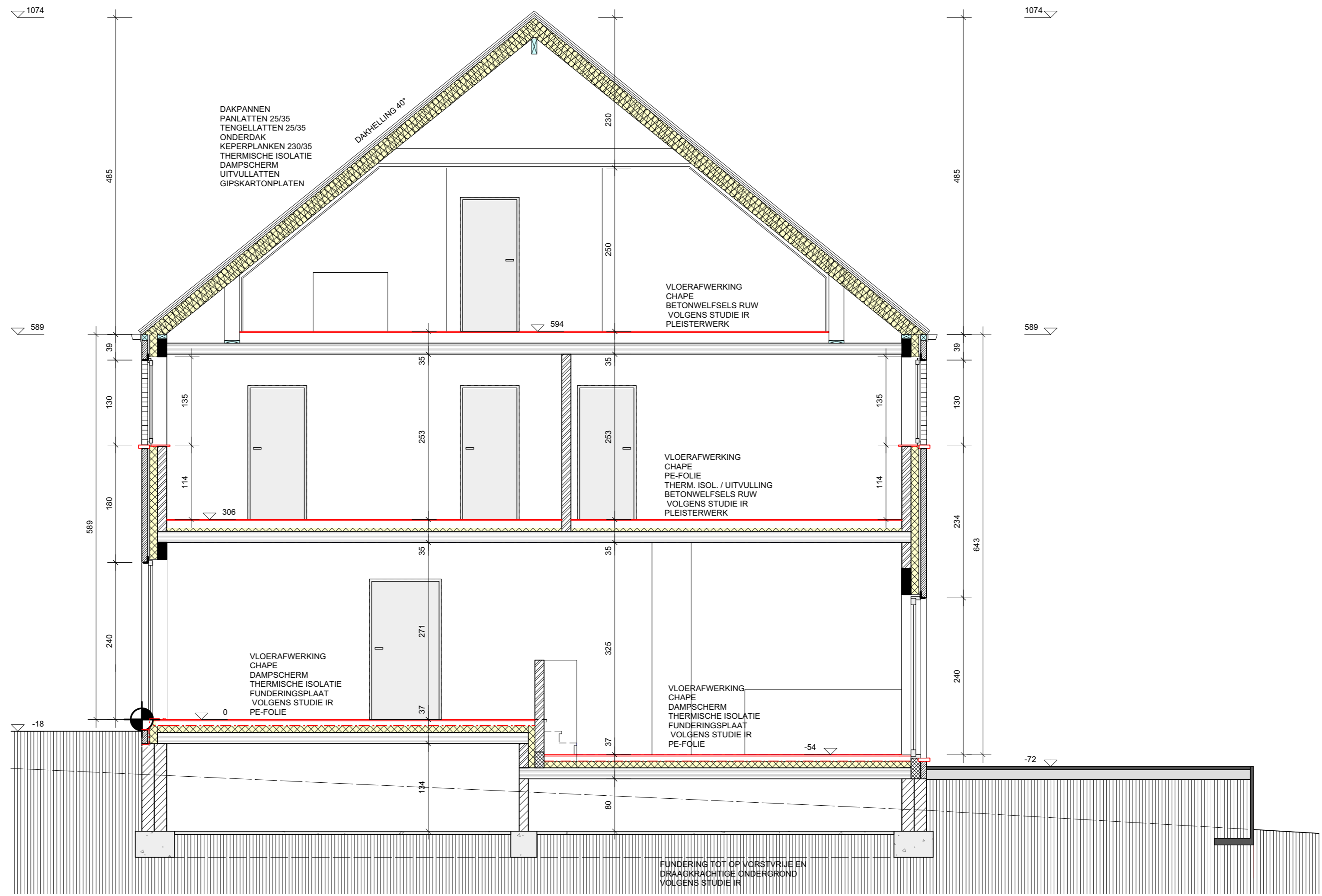
DOORSNEDE AA SCHAAL 1/50
