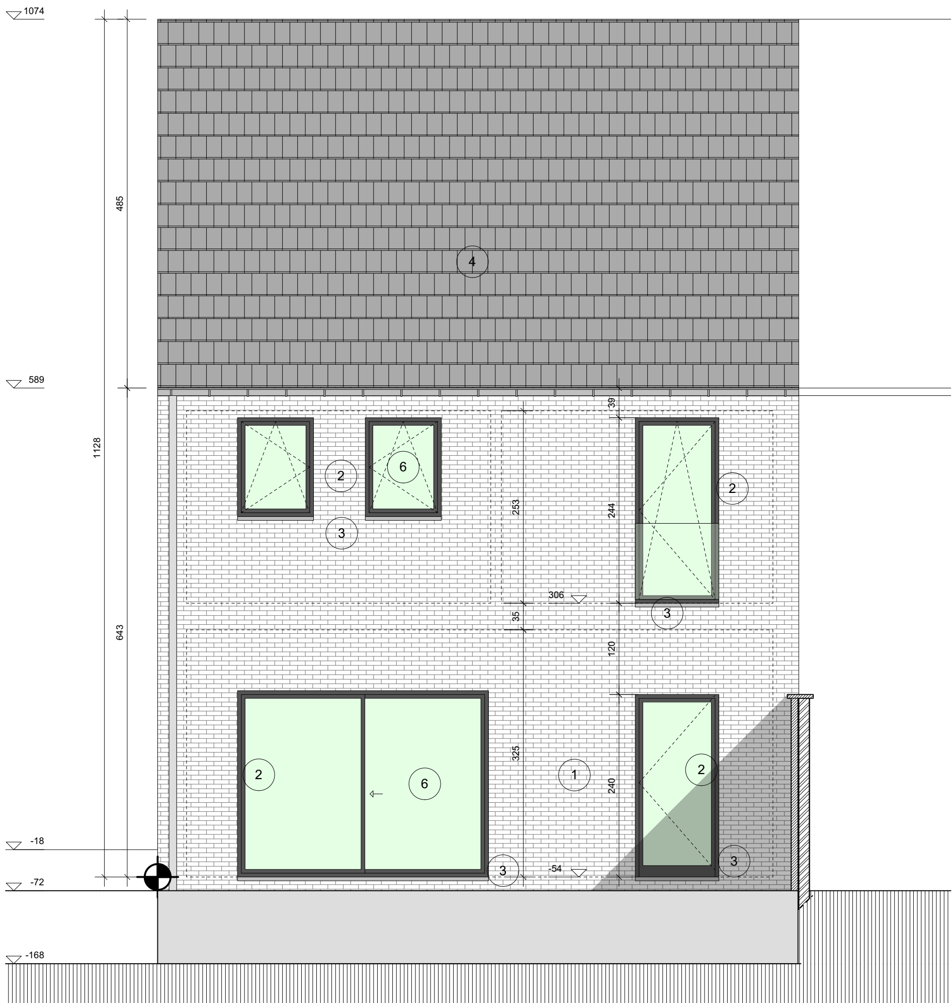
ACHTERGEVEL SCHAAL 1/50 0 50 100 cm
