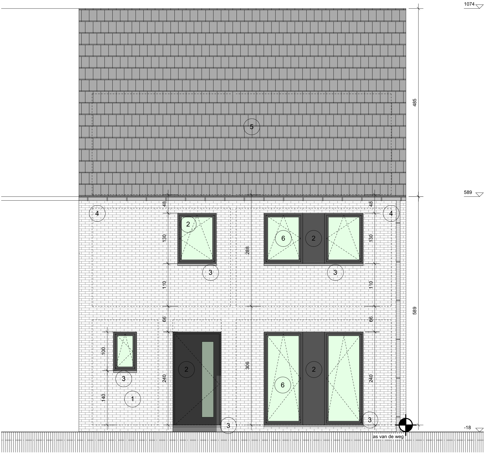
VOORGEVEL SCHAAL 1/50 0 50 100 cm
